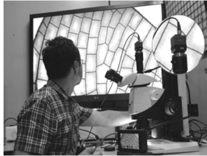
〈광학현미경시스템 개선〉 3D 촬영장비인 SYNACAM 광학현미경 접목활용
